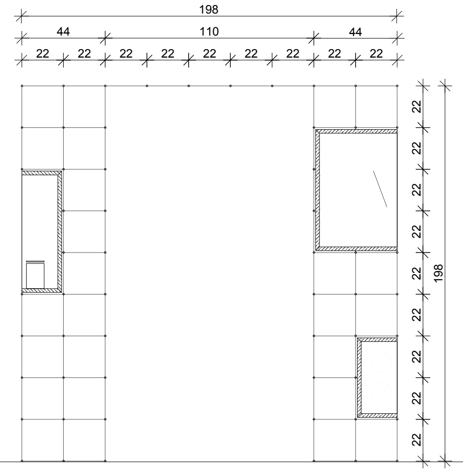
PRESJEK AA
